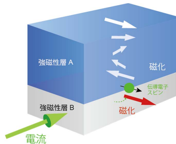
図：強磁性層 A および B から構成され「ねじれ磁気構造」を示す積層膜におけるスピントルクの模式図。
