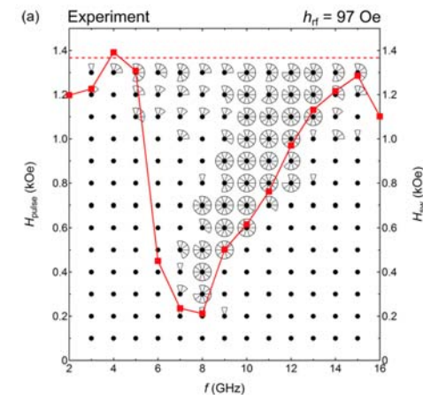
図1:パルス状の高周波磁場により評価した磁化スイッチング条件の磁場と周波数に対するマッピング。赤線は、高周波磁場を印加した状態で評価したスイッチング磁場である。
