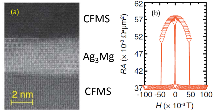
図 (a) Co_2Fe_{0.4}Mn_{0.6}Si (CFMS)/ Ag_3Mg /CFMS積層膜の高角散乱環状暗視野走査透過顕微鏡(HAADF-STEM)像。 Ag_3Mg 層部分に L1_2 相に起因する周期的なコントラストが確認できる。(b) 作製したCPP-GMR素子の磁気抵抗曲線。発表論文[1] ©IOP Publishing 2017.
